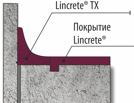
Примыкание к наружной стене
